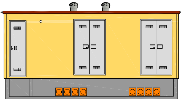
PROSPETTO FRONTALE
