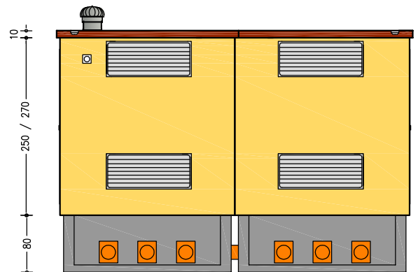
PROSPETTO DESTRO
